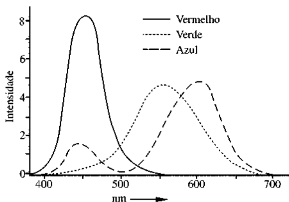
Figura 1. Espectros correspondentes às cores vermelho, verde e azul.
