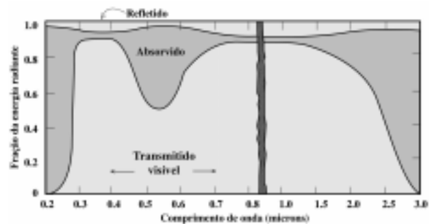
Figura 5. Variações da reflexão, absorção e transmissão com o comprimento de onda de uma luz branca incidindo sobre um vidro verde (adaptado da referência 7).
