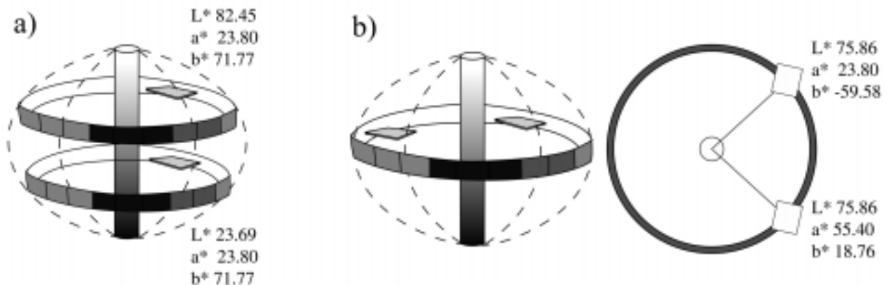
Figura 8. Representação de algumas cores através do Sistema Cielab (adaptado da referência 1).
