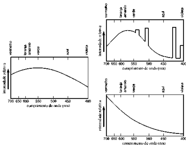
Figura 4. Distribuição de comprimentos de onda para diferentes fontes de iluminação (adaptado da referência 1).
