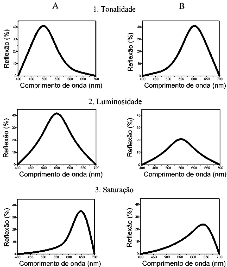
Figura 6. Elementos que determinam a cor de um objeto (adaptado da referência 1).
