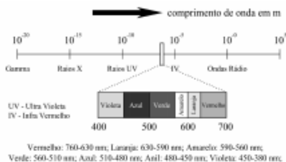
Figura 3. Representação do espectro eletromagnético com destaque para a região visível.
