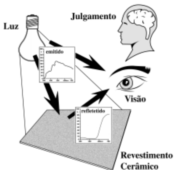
Figura 2. Representação esquemática da percepção da cor por um observador (adaptado da referência 1).
